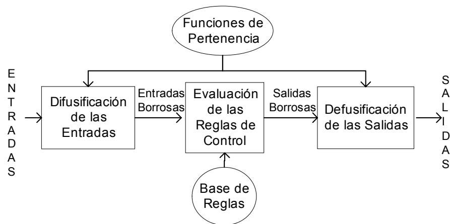
Figura 3. Sistema de inferencia difusa
