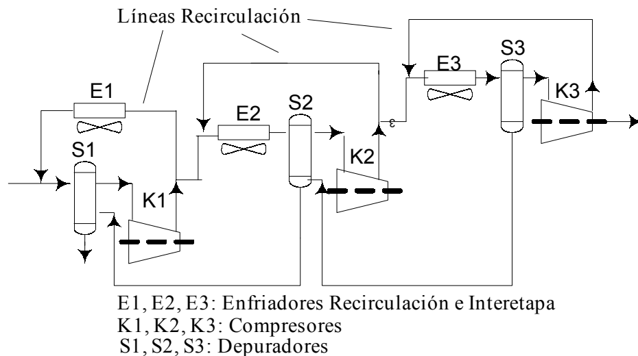
Figura 1. Diagrama esquemático de un tren de compresión
